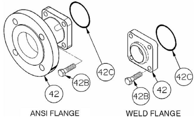
ANSI FLANGE
